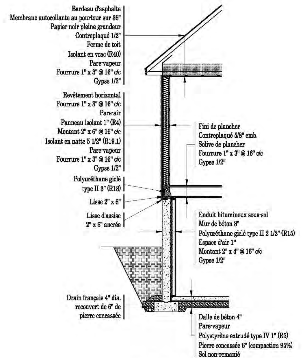
Coupe de mur typique Echelle: aucune
