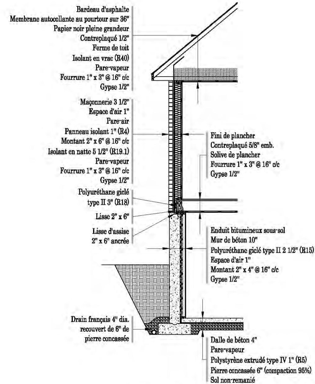
Coupe de mur typique Echelle: aucune
