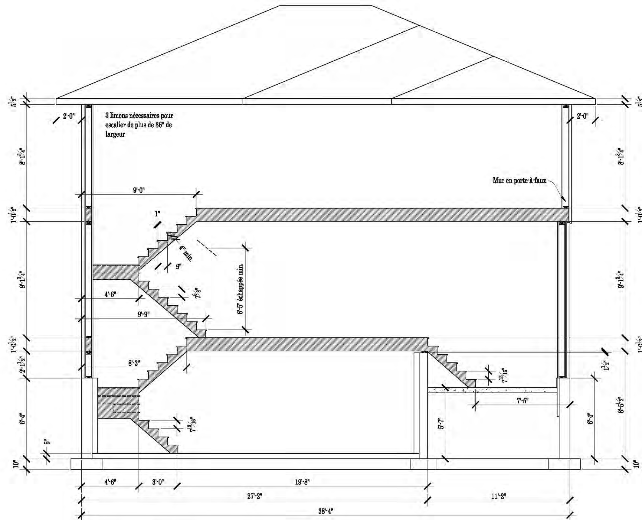
Coupe C (escalier)
